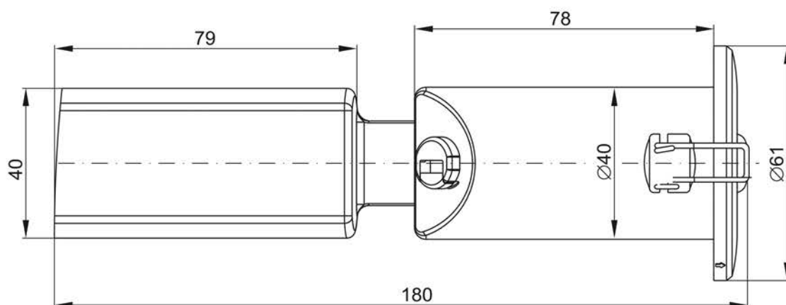
Рисунок 1 – ДПА 060
