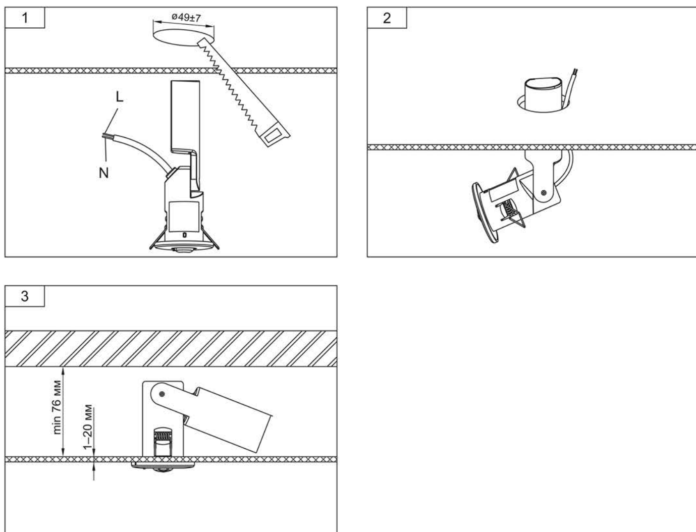
Рисунок 5 – Монтаж ДПА 060
