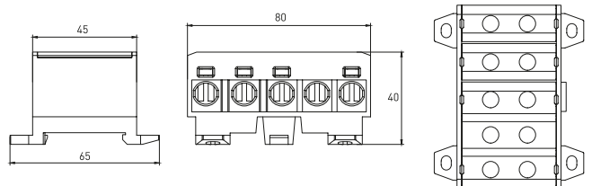
КСВ 2,5-35 (пятиполюсные)
