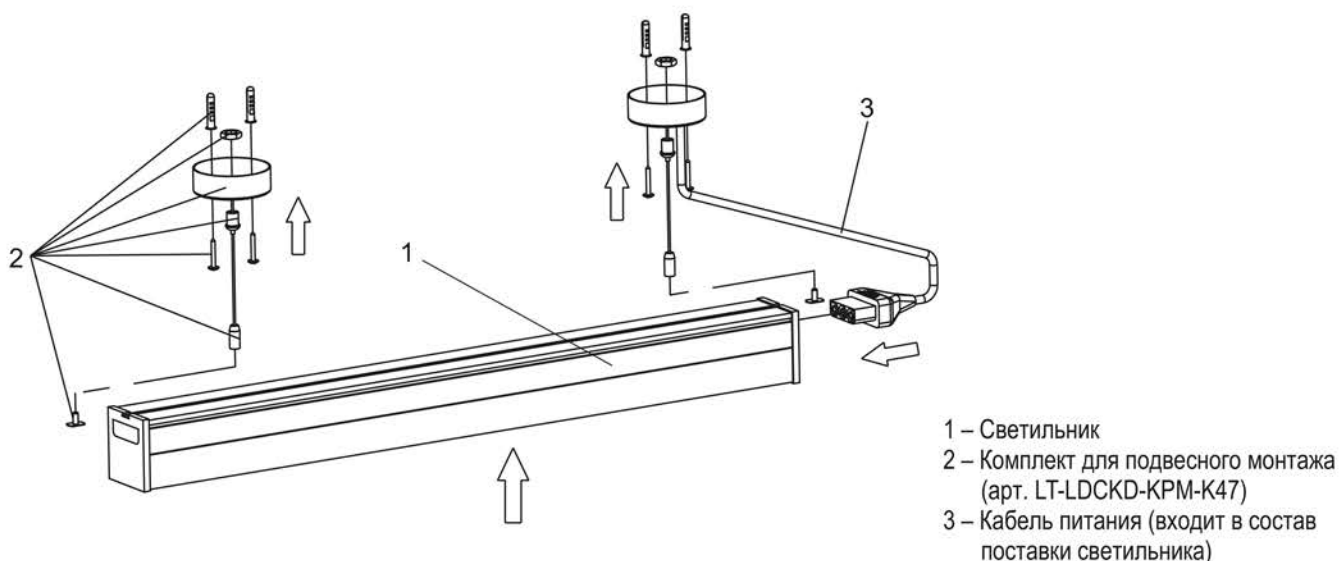
Рисунок 6 – Подвесной монтаж светильника на тросе
