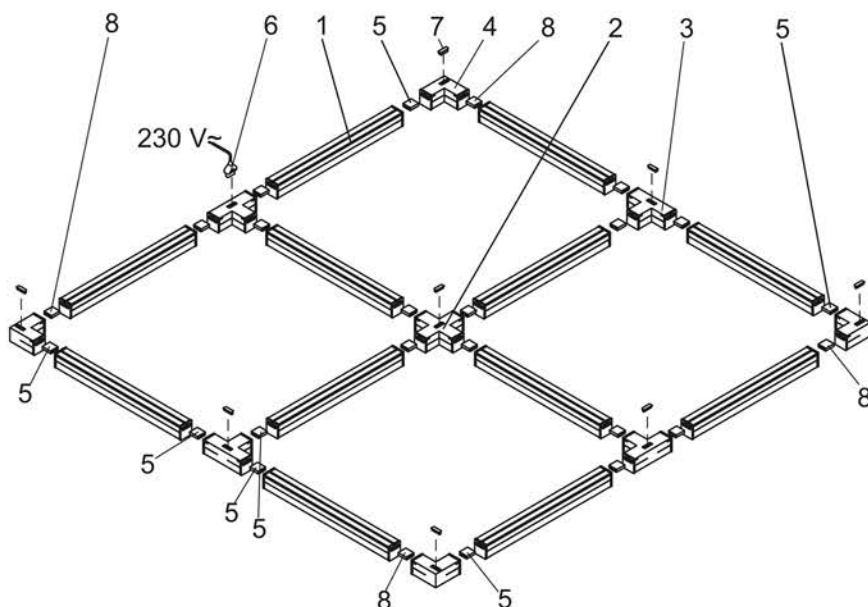
Рисунок 10 – Монтаж и подключение к сети 230 В группы квадратных систем магистральных светильников 1010
