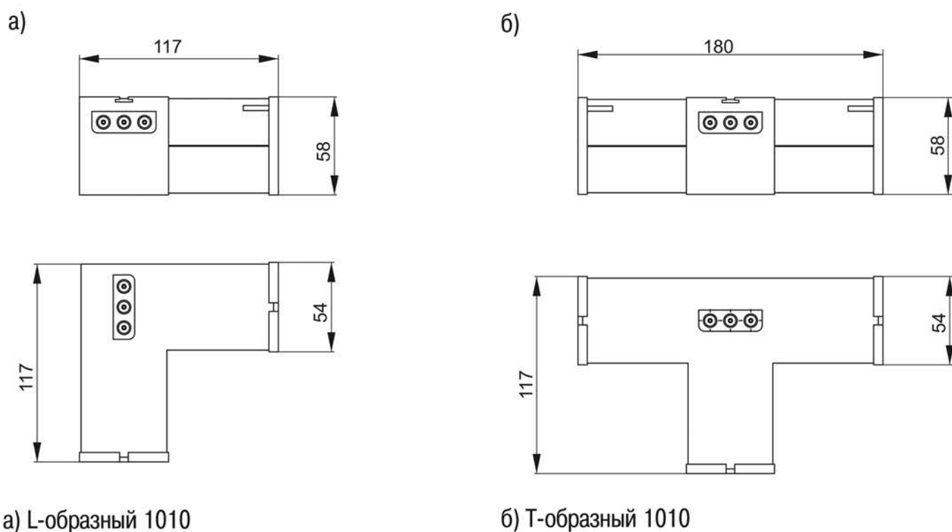
Рисунок 2 – Габаритные размеры светильника 1010 (лист 1 из 2)
