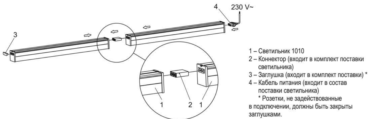
Рисунок 8 – Монтаж и подключение к сети 230 В линейной системы магистральных светильников 1010
