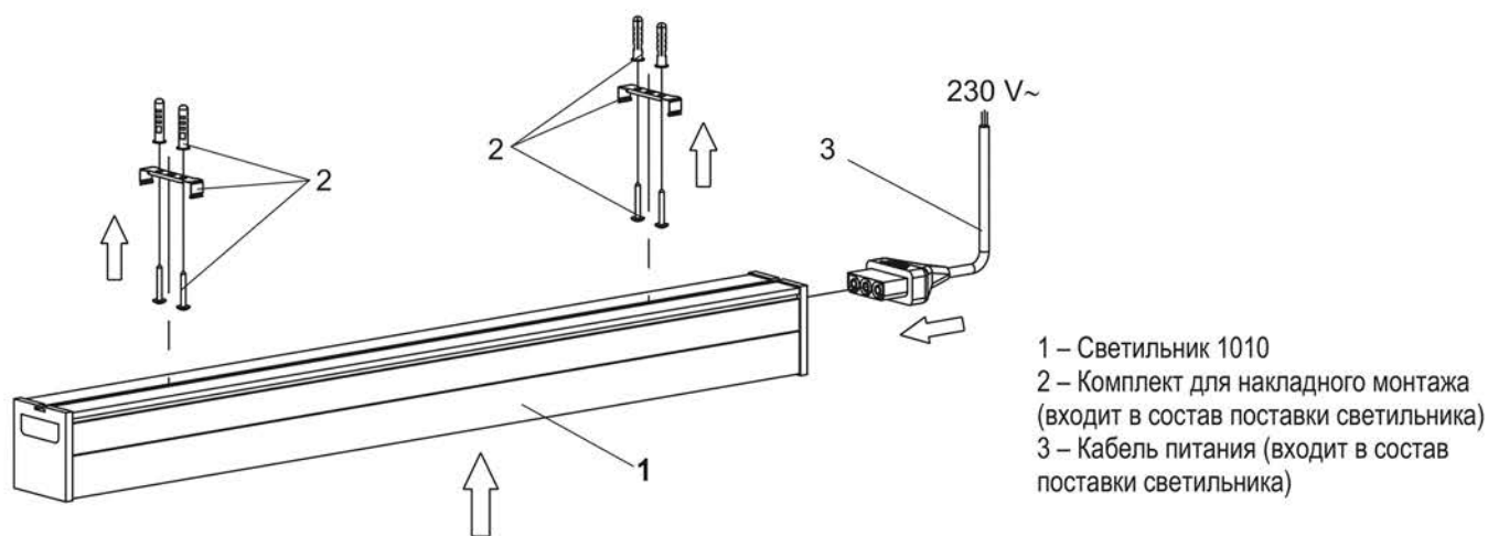
Рисунок 3 – Накладной монтаж магистрального светильника 1010 и подключение к сети 230 В
