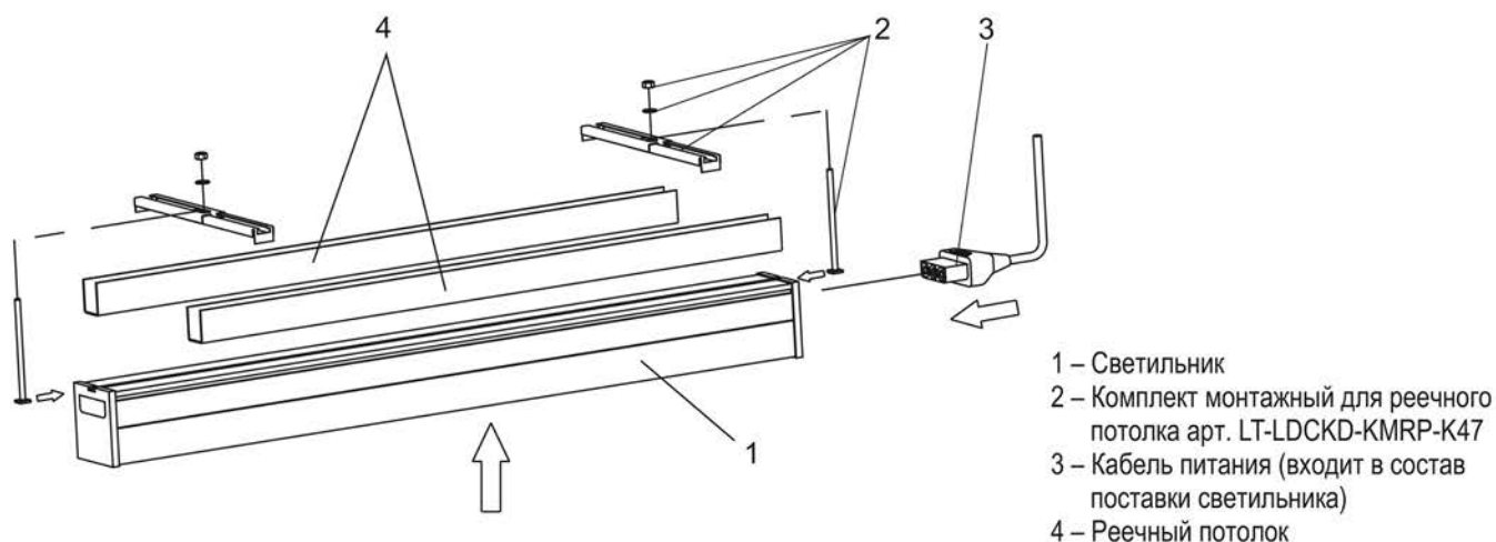
Рисунок 5 – Монтаж светильника на реечный потолок
