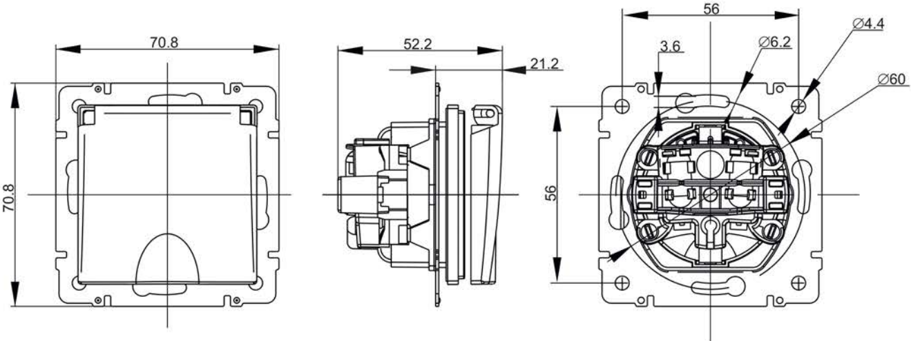
ж) РС6ш10-3-44-БрХ*; РС6ш10-3-БрХ*
