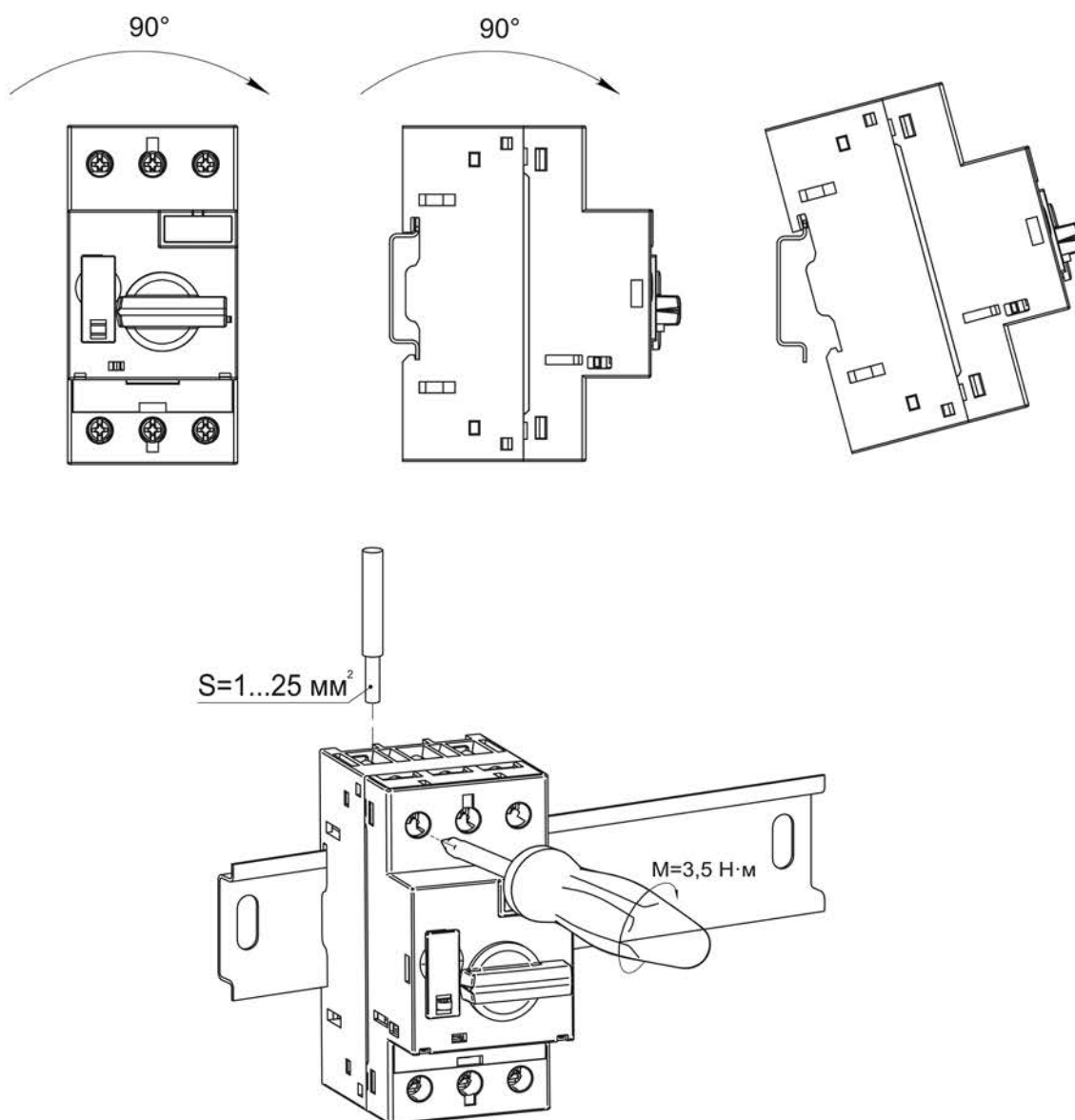
Рисунок 9 – Монтаж выключателя
