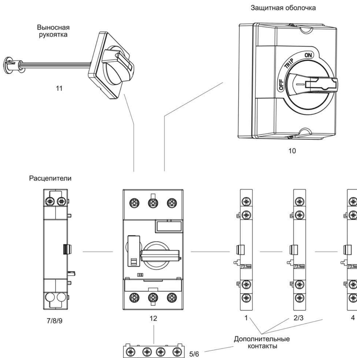
Рисунок 8 – Разнесенная сборка
