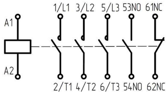
Рисунок Б.4 – Контакторы типа LC1E120-E630
