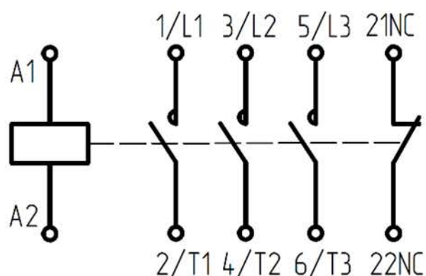
Рисунок Б.2 – Контакторы типа LC1E0901-E3201
