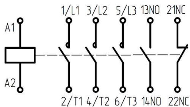
Рисунок Б.3 – Контакторы типа LC1E40-E95
