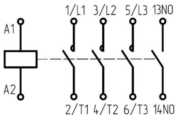
Рисунок Б.1– Контакторы типа LC1E0910-E3210
