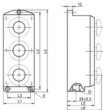
Рисунок А.1 – Габаритные и установочные размеры постов для установки в нишу
