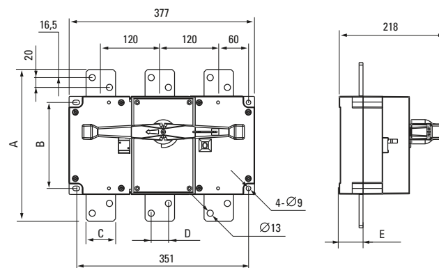
Выключатель PowerSwitch 1000-1600 А
