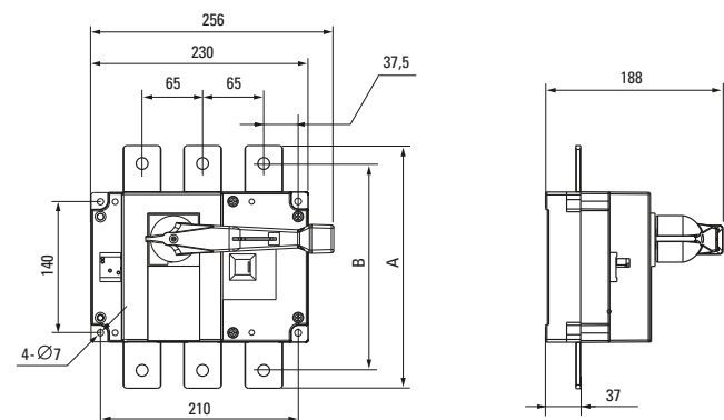
Выключатель PowerSwitch 400-630 А
