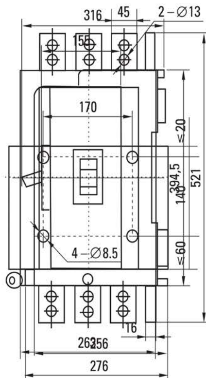
Габаритные и установочные размеры ВА-99М 1250А
