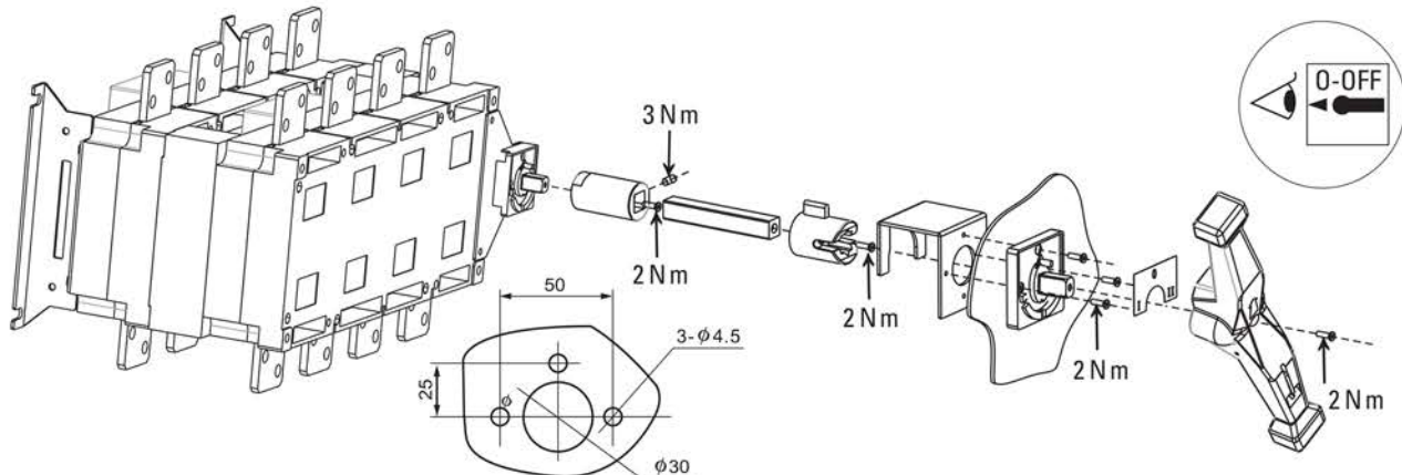
Рисунок 9 - Монтаж ручки на дверцу шкафа
