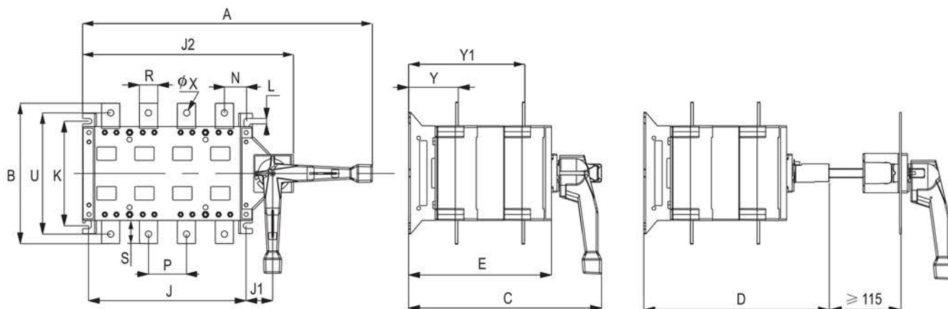
Рисунок 1 - Монтажные размеры рубильников 63 А - 630 А
