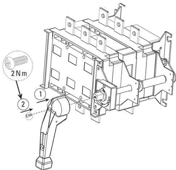
Рисунок 7 - Монтаж ручки на корпус рубильников
