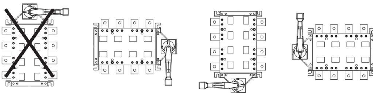
Рисунок 7 - Рабочее положение рубильников при эксплуатации
