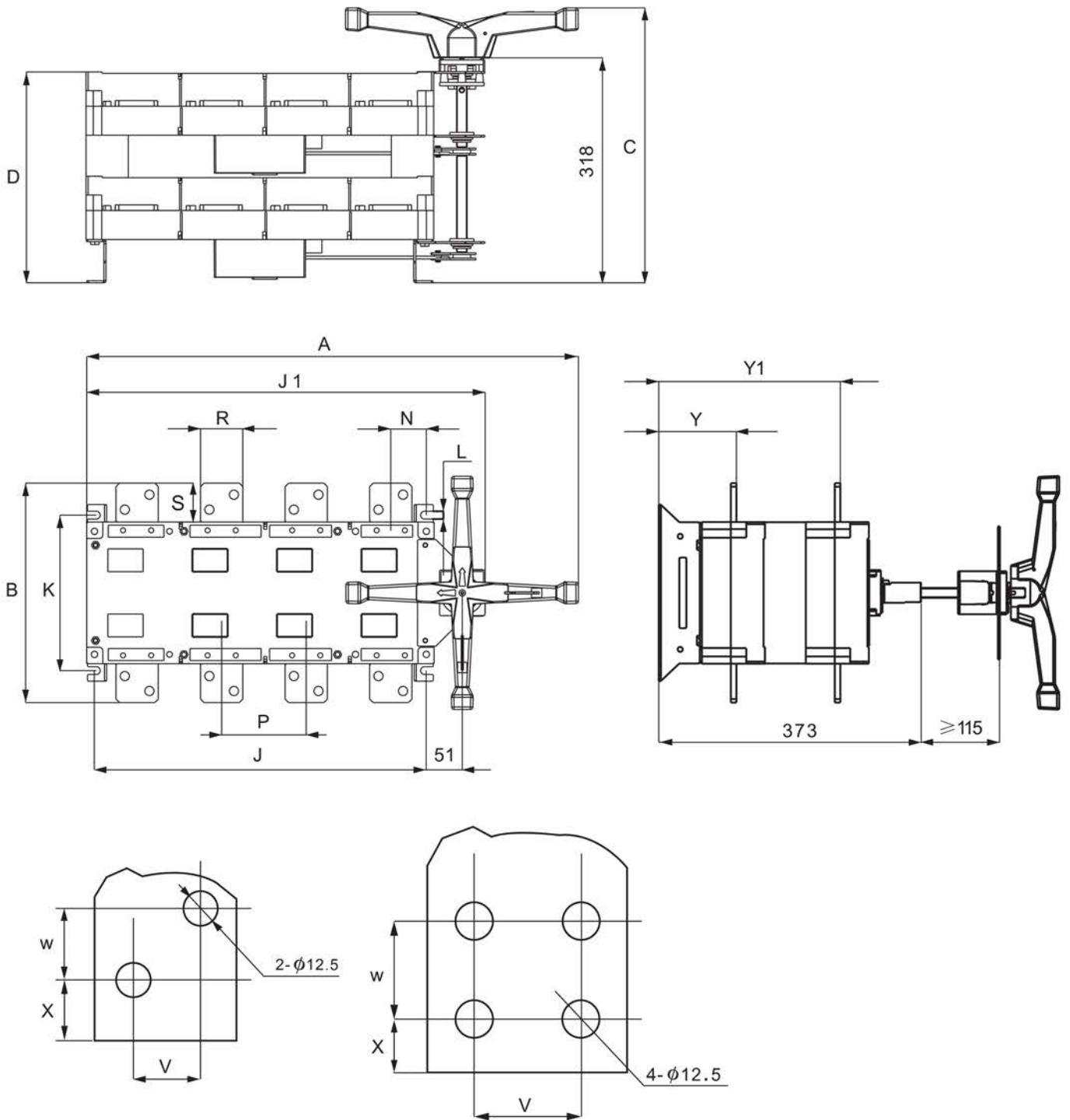
Рисунок 2 - Монтажные размеры рубильников 1000 А - 1600 А
