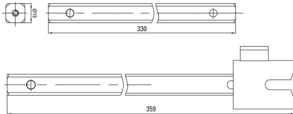
Рисунок 5 - Габаритные размеры штока
