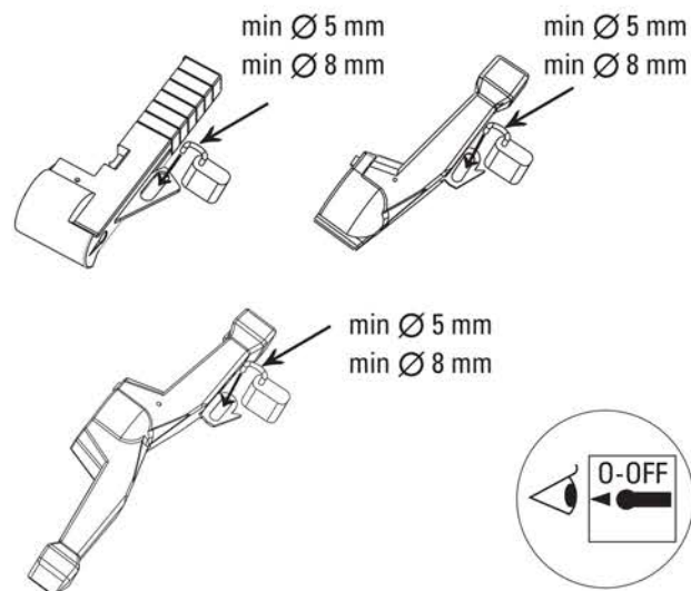
Рисунок 8 - Блокировка ручки навесным замком
