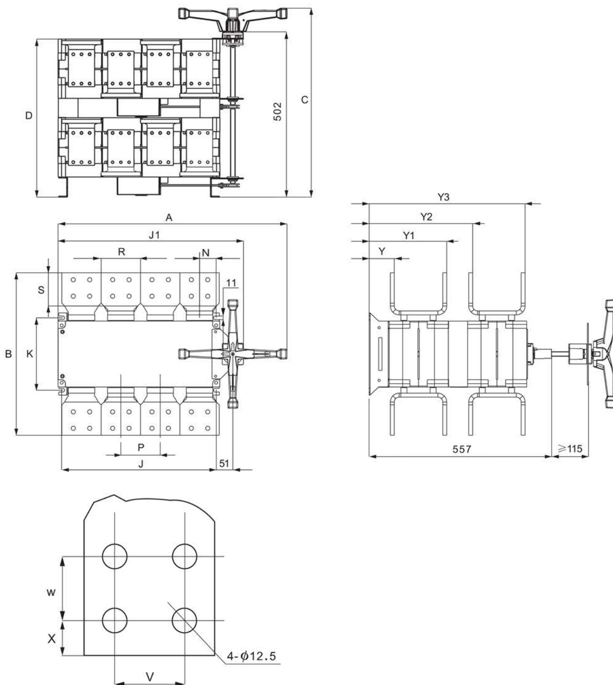
Рисунок 4 - Монтажные размеры рубильников 3150 А
