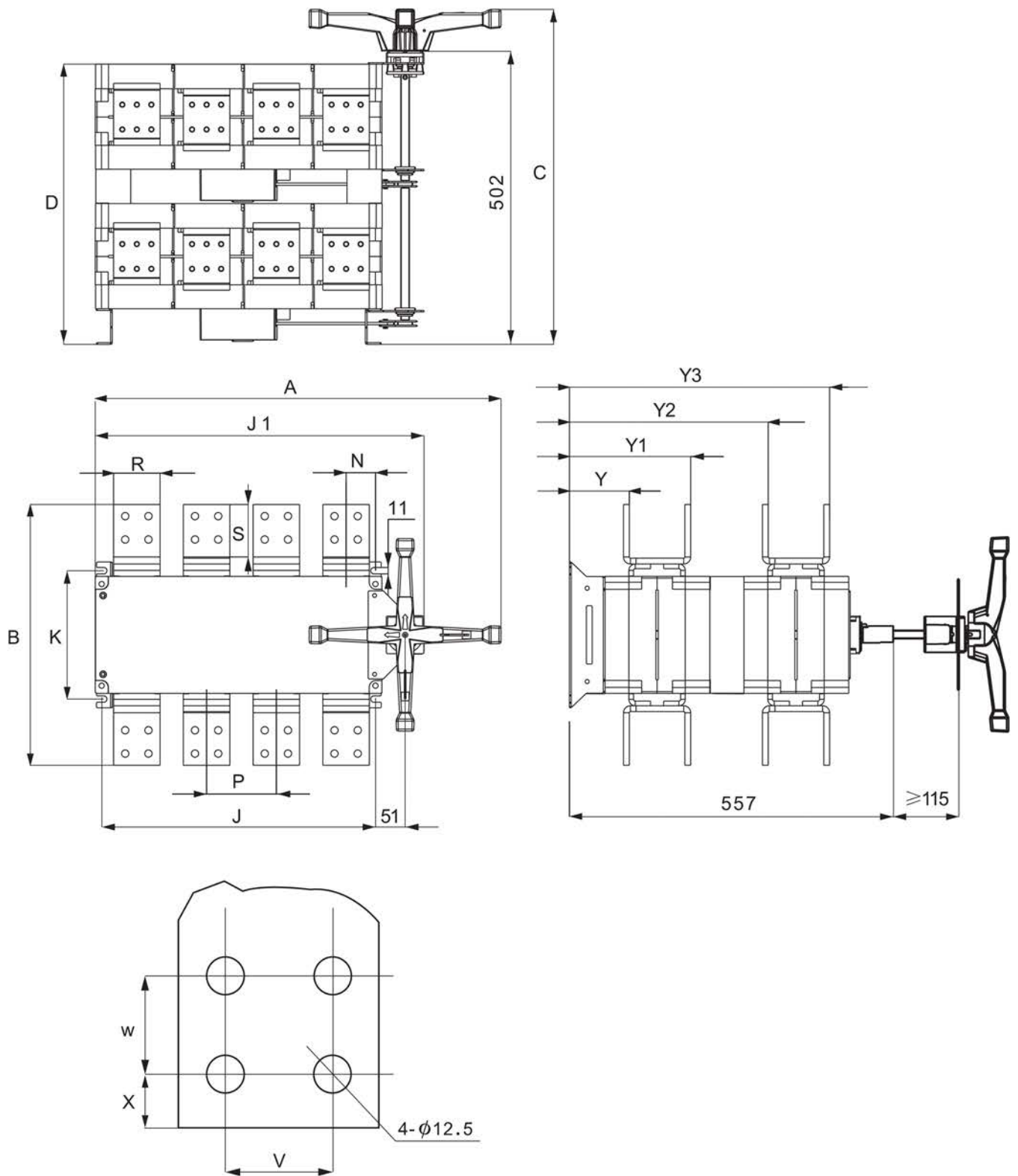
Рисунок 3 - Монтажные размеры рубильников 2000 А - 2500 А
