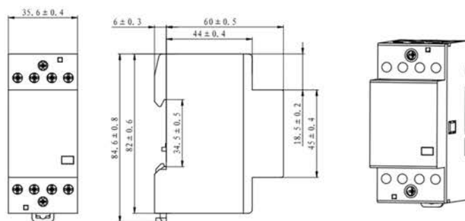
Рисунок Б.2 – Габаритные, установочные и присоединительные размеры OptiDin MK-100-25..., OptiDin MK-100-63...
