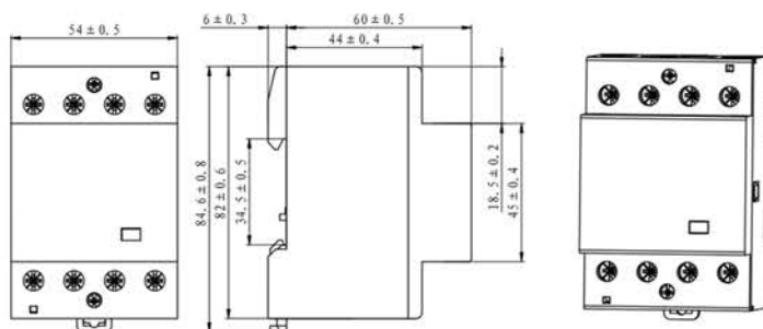
Рисунок Б.3 – Габаритные, установочные и присоединительные размеры OptiDin MK-100-63..., OptiDin MK-100-80..., OptiDin MK-100-100...
