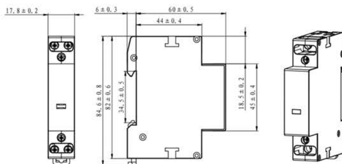
Рисунок Б.1 – Габаритные, установочные и присоединительные размеры OptiDin MK-100-20..., OptiDin MK-100-RC-R-230AC
