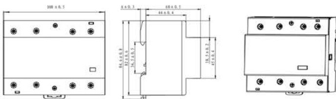
Рисунок Б.4 - Габаритные, установочные и присоединительные размеры OptiDin MK-100-80..., OptiDin MK-100-100...
