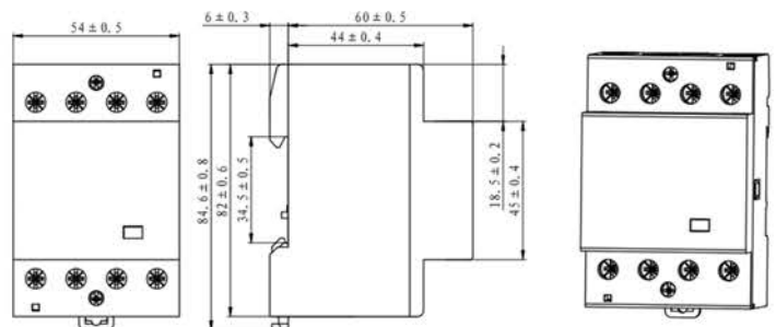
Рисунок Б.3 - Габаритные, установочные и присоединительные размеры OptiDin МК-100-63..., OptiDin МК-100-80..., OptiDin МК-100-100...
