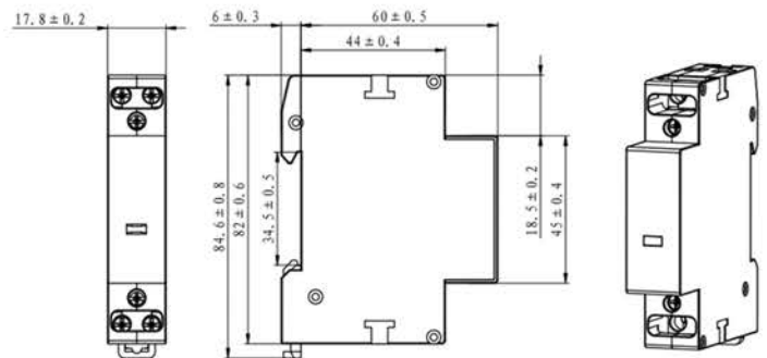
Рисунок Б.1 - Габаритные, установочные и присоединительные размеры OptiDin МК-100-20..., OptiDin МК-100-RC-R-230АС
