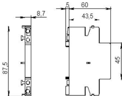
Рисунок Б.5 - Габаритные, установочные и присоединительные размеры OptiDin MK 11
