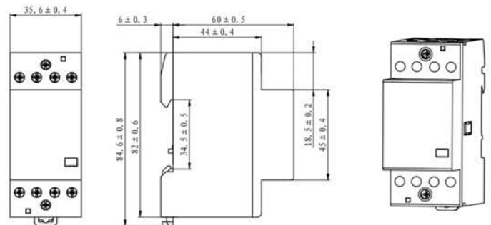
Рисунок Б.2 - Габаритные, установочные и присоединительные размеры OptiDin МК-100-25..., OptiDin МК-100-63...
