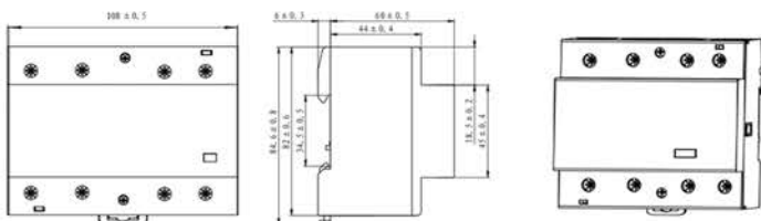
Рисунок Б.4 - Габаритные, установочные и присоединительные размеры OptiDin MK-100-80..., OptiDin MK-100-100...
