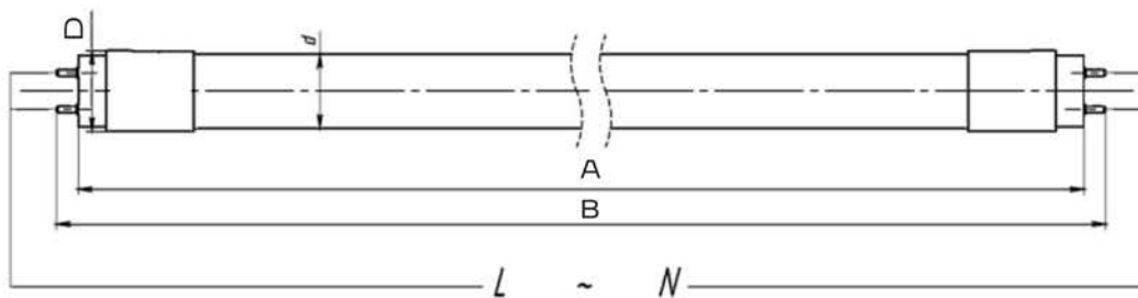
Рис. 1. Общий вид, основные размеры и схема подключения ламп.
