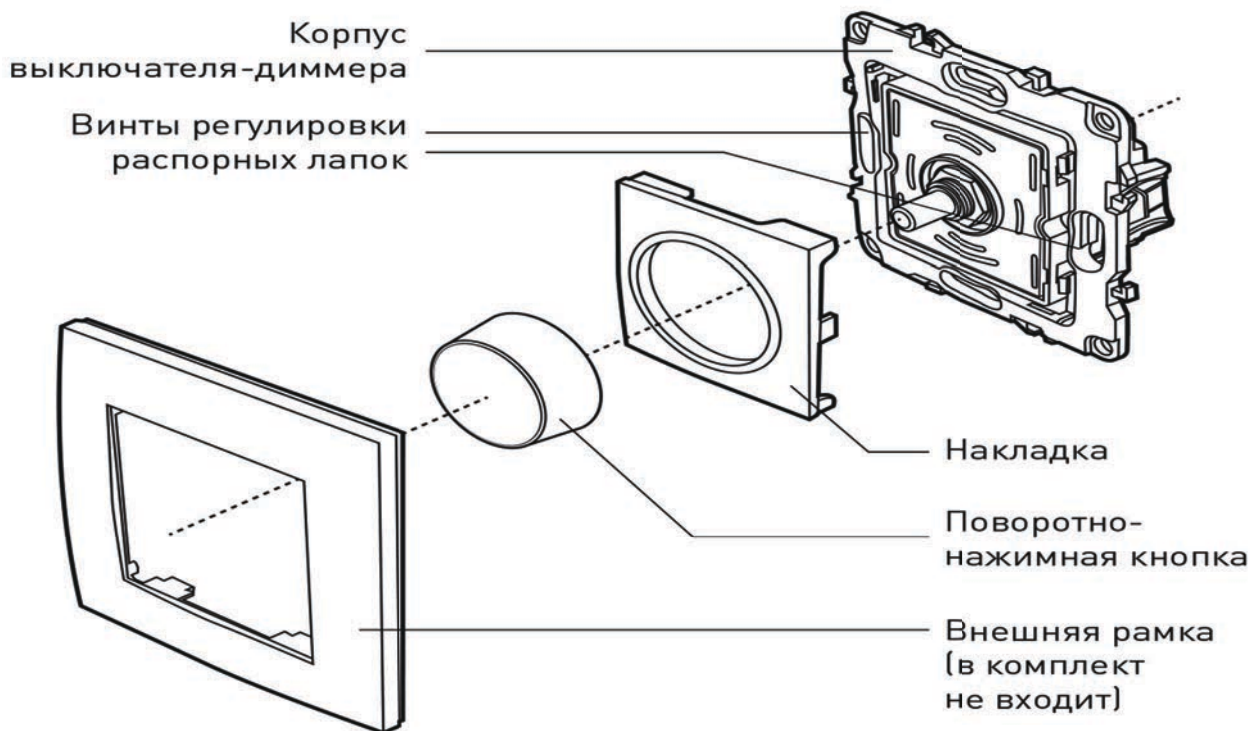
Рис.2 Монтаж выключателя-диммера ЭРА.
