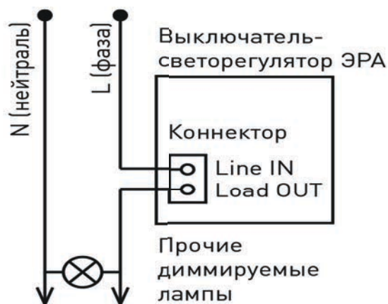
Рис.1 Схема подключения изделия.
