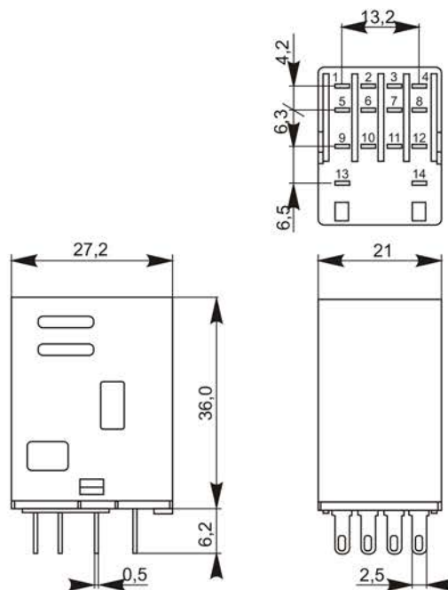
б) реле интерфейсное / b) interface relay / б) интерфейс релесі ORM-1-4C-DC24V-L-B, ORM-1-4C-AC220V-L-B
