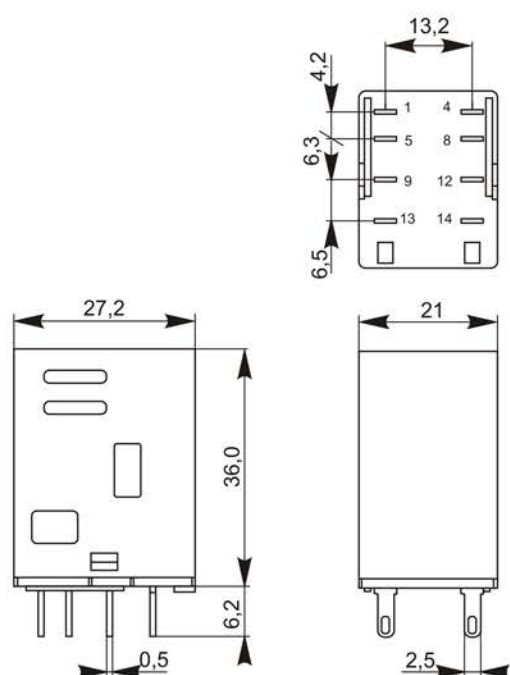
а) реле интерфейсное / interface relay / интерфейс релесі ORM-1-2C-DC24V-L-B, ORM-1-2C-AC220V-L-B
