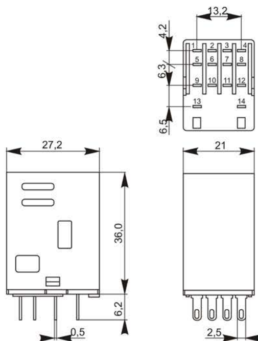
б) реле интерфейсное / b) interface relay / б) интерфейс релесі ORM-1-4C-DC24V-L-B, ORM-1-4C-AC220V-L-B
