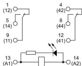
а) схема реле интерфейсного / diagram of the interface relay / интерфейс релесінің схемасы ORM-1-2C-DC24V-L-B, ORM-1-2C-AC220V-L-B
