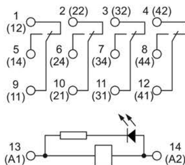
б) реле интерфейсное / b) interface relay / б) интерфейс релесі ORM-1-4C-DC24V-L-B, ORM-1-4C-AC220V-L-B
