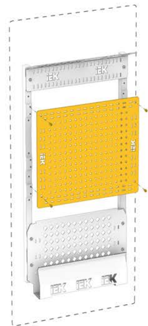
2.1 Установка монтажной панели Installation of mounting panel
