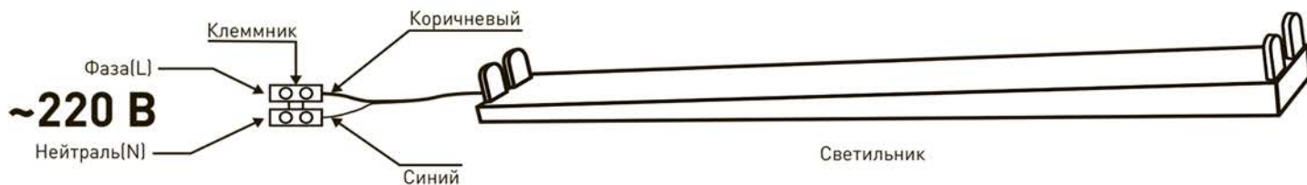
Рис.1. Схема подключения светильника к сети 220В.
