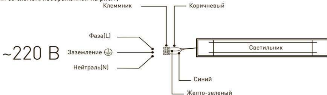
Рис.1. Схема подключения светильника к сети 220В.
