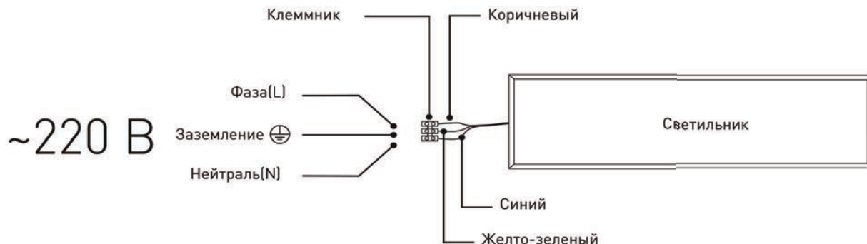
Рис.1. Схема подключения светильника к сети 220В.
