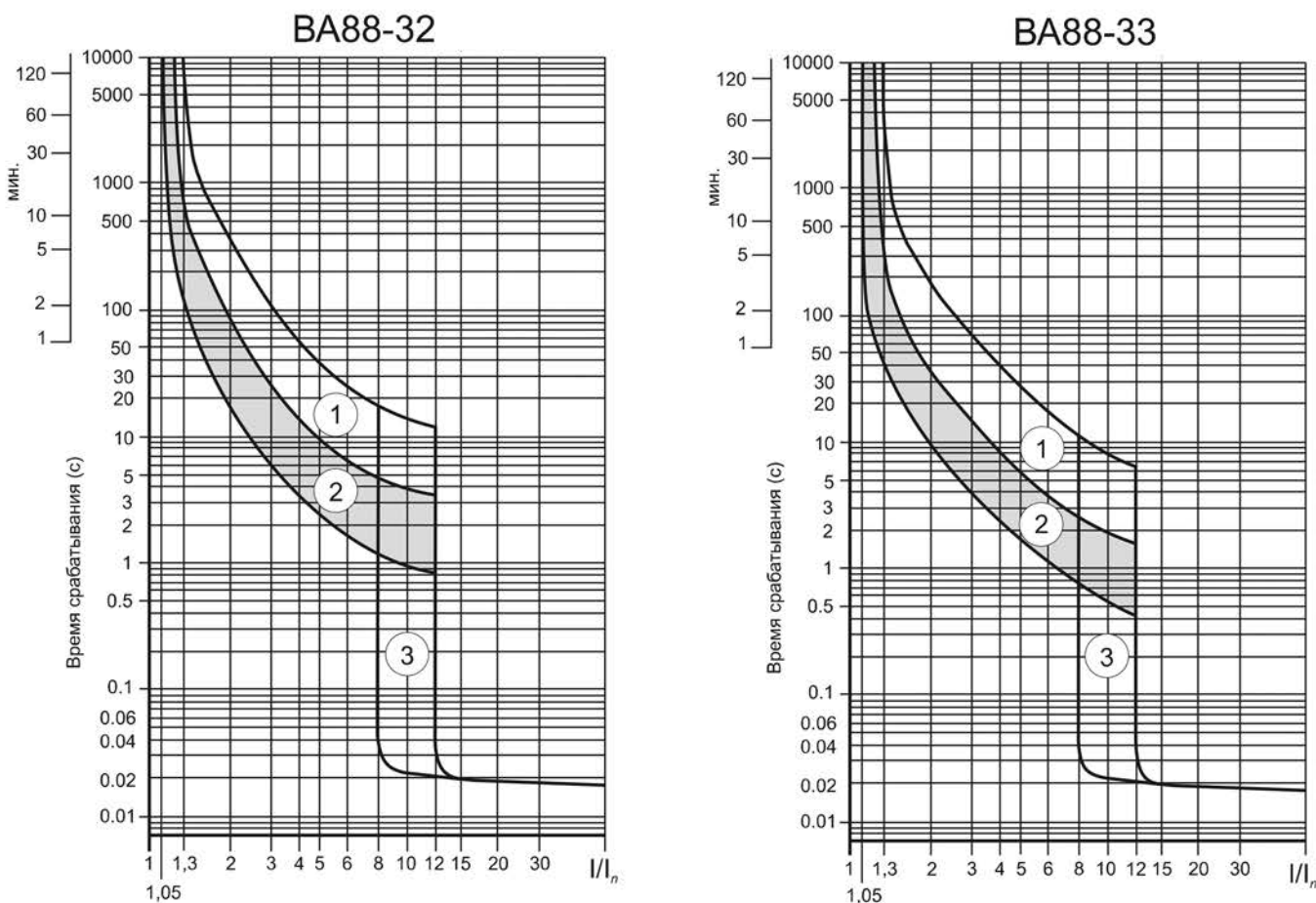
Рисунок 1 – Время-токовые характеристики выключателей ВА88-32 и ВА-33
