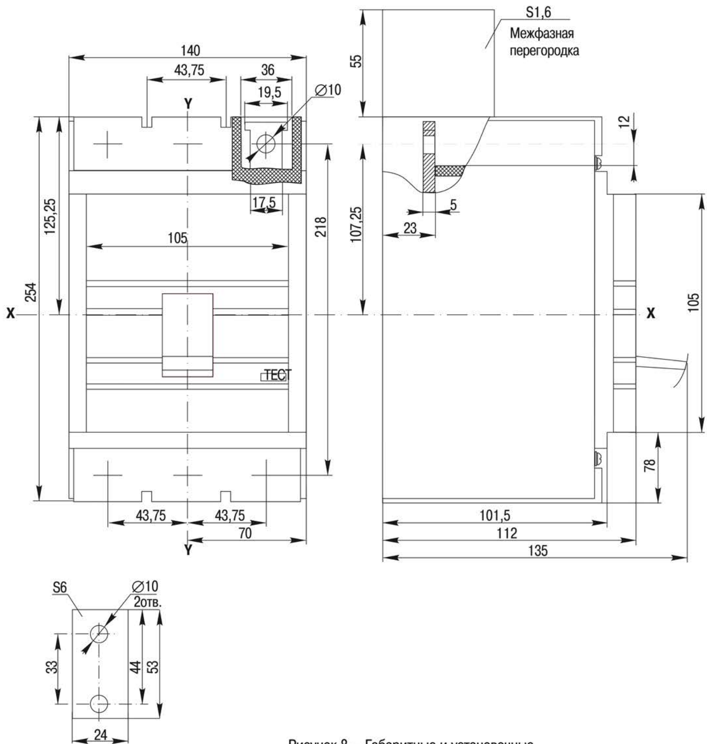
Рисунок 8 – Габаритные и установочные размеры выключателя ВА88-37
