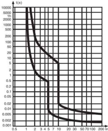
Рис. 2. Время-токовая характеристика С.
