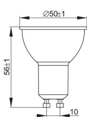
Рисунок 14 – Лампа LED PAR16, 8 Вт, 10 Вт цоколь GU10
