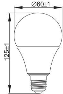
Рисунок 4 – Лампа LED A60, 20 Вт цоколь E27
