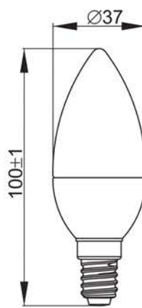
Рисунок 7 – Лампа LED C35, 8 Вт, 10 Вт, 12 Вт, цоколь E14
