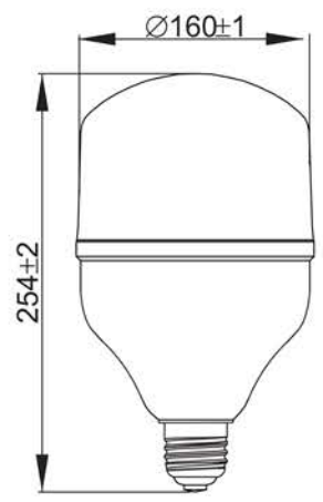
Рисунок 12 – Лампа LED HP, 70 Вт цоколь E27/E40
