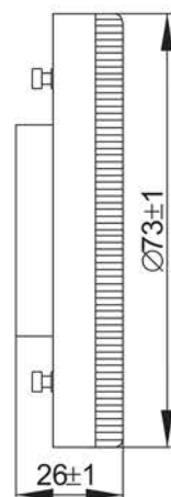
Рисунок 15 – Лампа LED T75, 8 Вт, 10 Вт цоколь GX53
