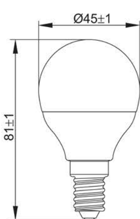
Рисунок 9 – Лампа LED G45, 8 Вт, 10 Вт, 12 Вт, цоколь E14
