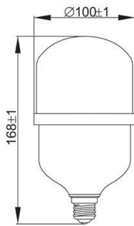
Рисунок 10 – Лампа LED HP, 30 Вт цоколь E27
