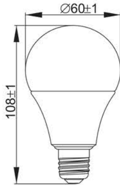
Рисунок 2 – Лампа LED A60, 11 Вт, 12 Вт цоколь E27
