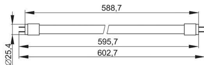
Рисунок 17 – Лампа LED T8, 10 Вт цоколь G13
