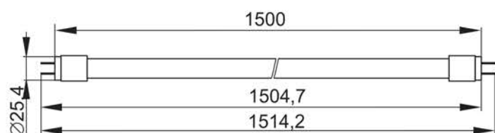
Рисунок 19 – Лампа LED T8, 25 Вт цоколь G13
