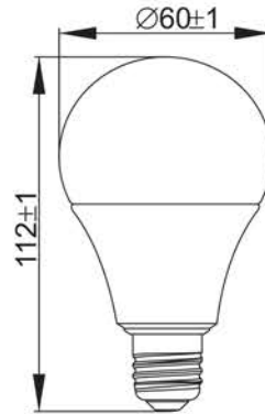
Рисунок 3 – Лампа LED A60, 15 Вт цоколь E27
