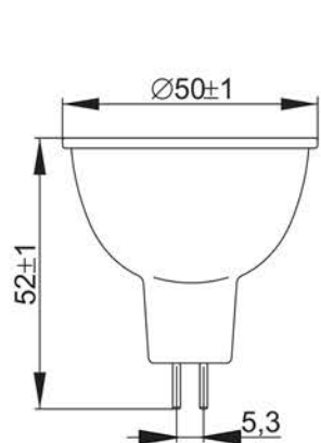
Рисунок 13 – Лампа LED MR16, 8 Вт, 10 Вт цоколь GU5.3
