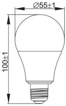
Рисунок 1 – Лампа LED A60, 8 Вт, 10 Вт цоколь E27
