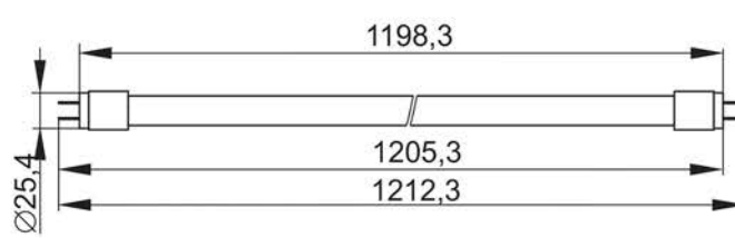
Рисунок 18 – Лампа LED T8, 20 Вт цоколь G13
