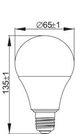
Рисунок 5 – Лампа LED A65, 25 Вт цоколь E27
