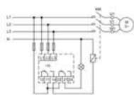
а) ORF-SP-130-650VAC Без функции контроля центральной линии
