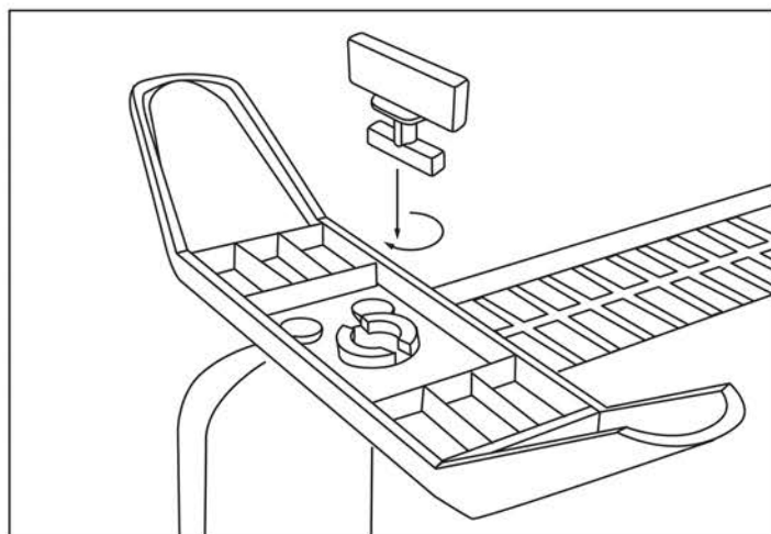
Рисунок 2. Установка опорных ножек
