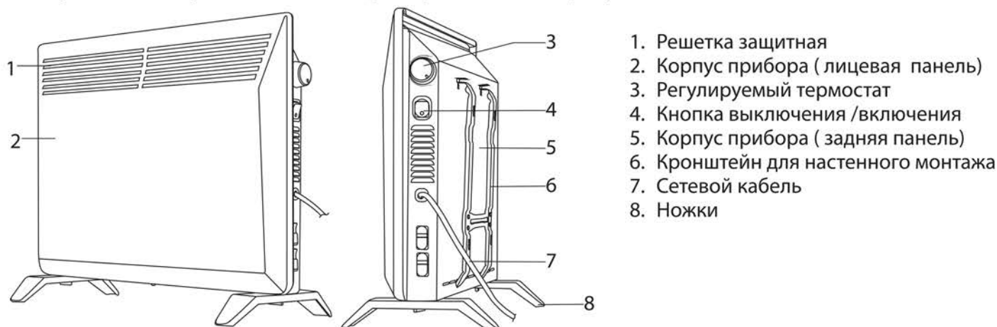
Рисунок 1. Устройство электрического конвектора
