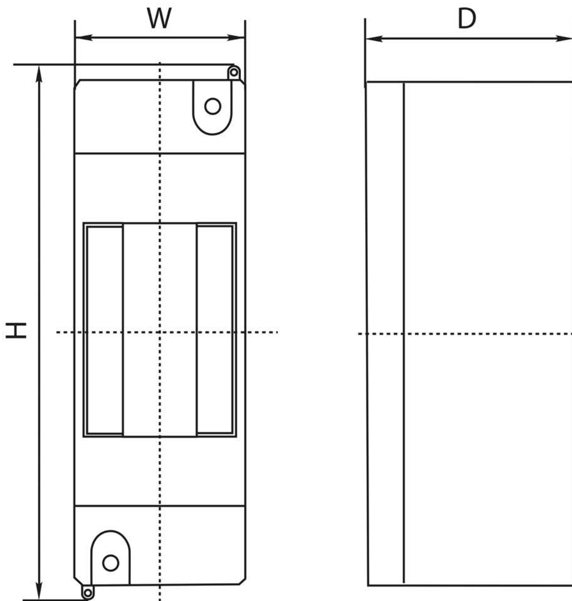
Рис. 1 - Габаритные размеры корпусов КМПн
