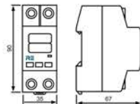
Габаритные размеры
