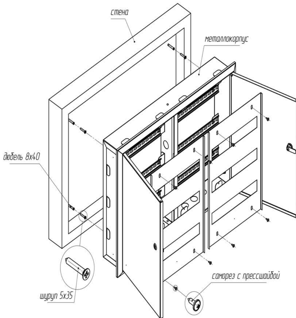
Рис. 1. Схема монтажа
