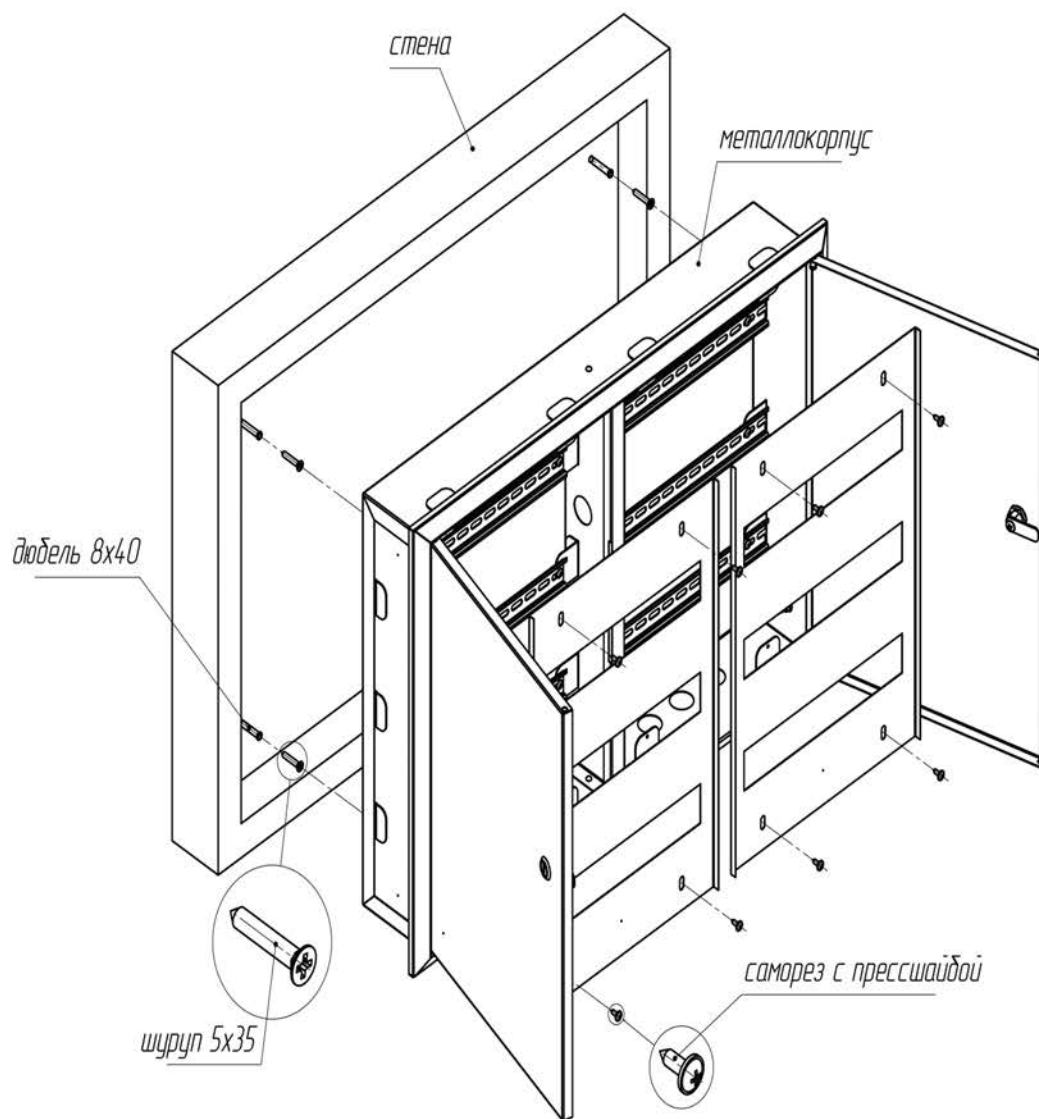
Рис. 1. Схема монтажа
