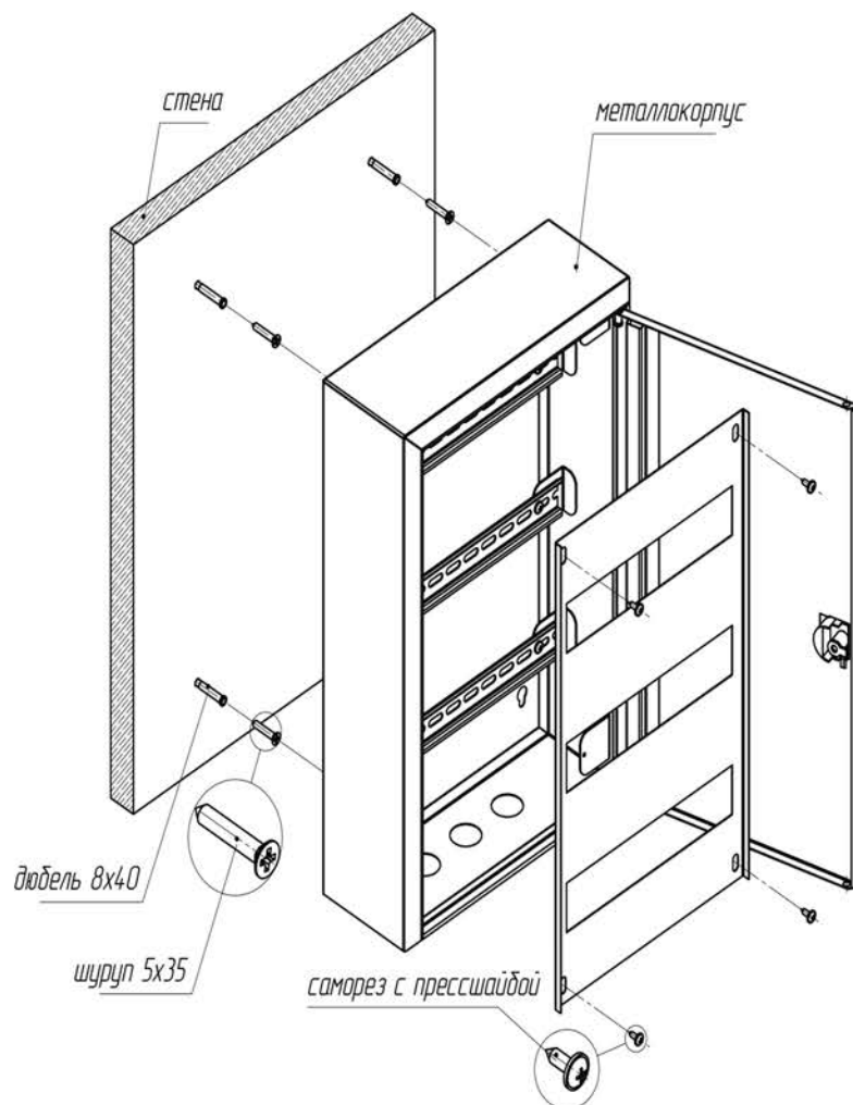
Рис. 1 - Схема монтажа
