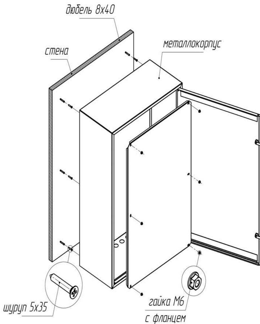
Рис. 1. Схема монтажа
