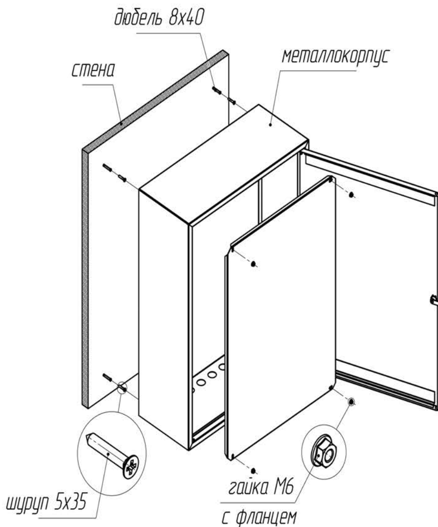
Рис. 1. Схема монтажа
