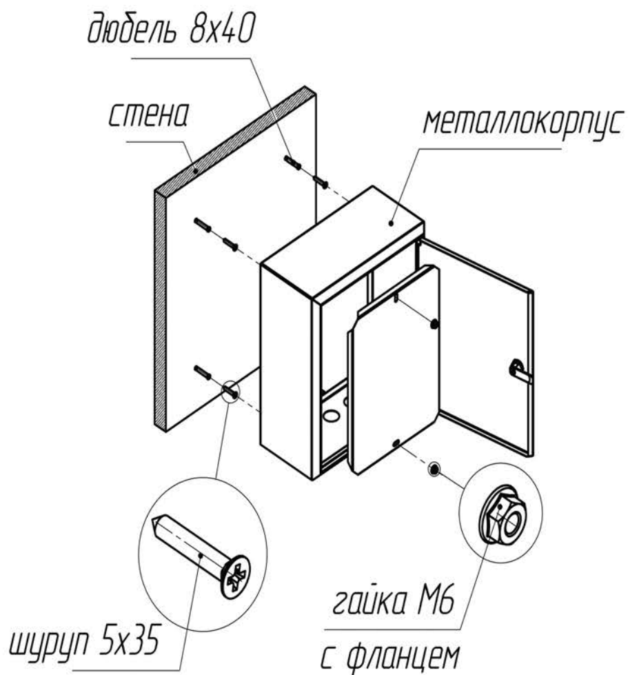
Рис. 1. Схема монтажа
