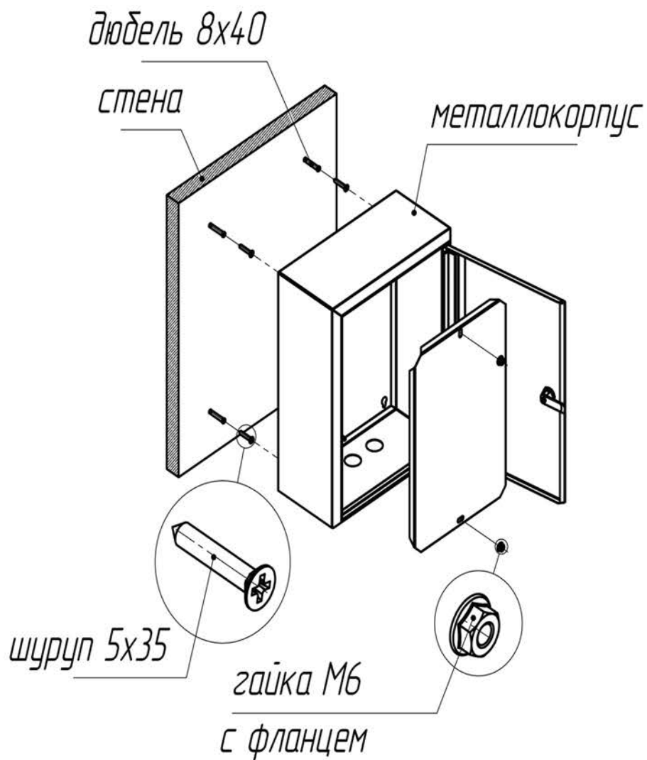
Рис. 1. Схема монтажа
