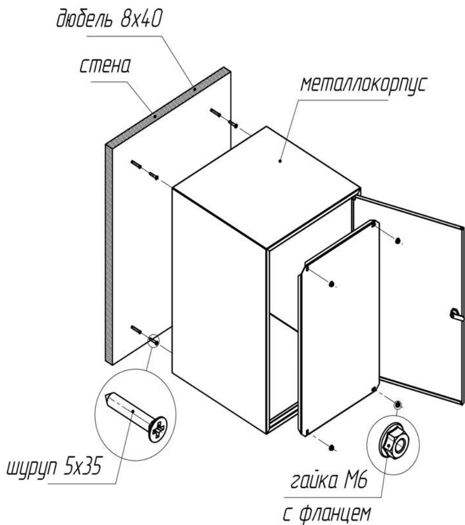
Рис. 1. Схема монтажа
