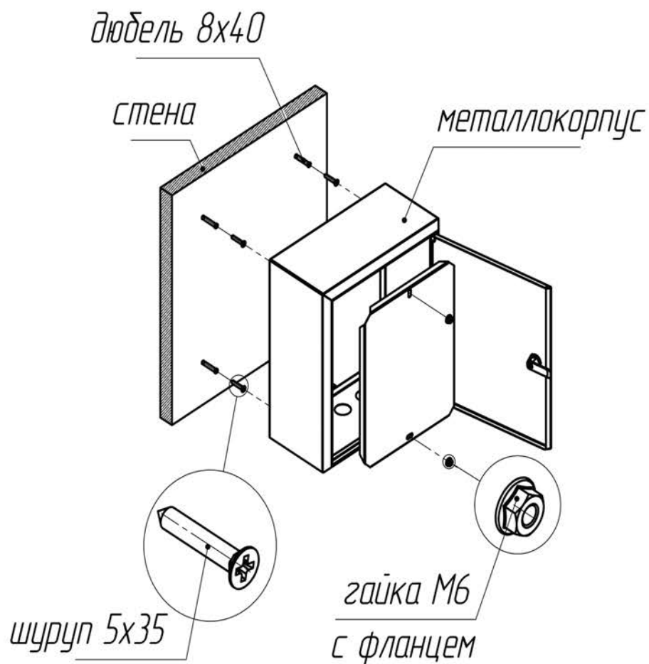
Рис. 1. Схема монтажа
