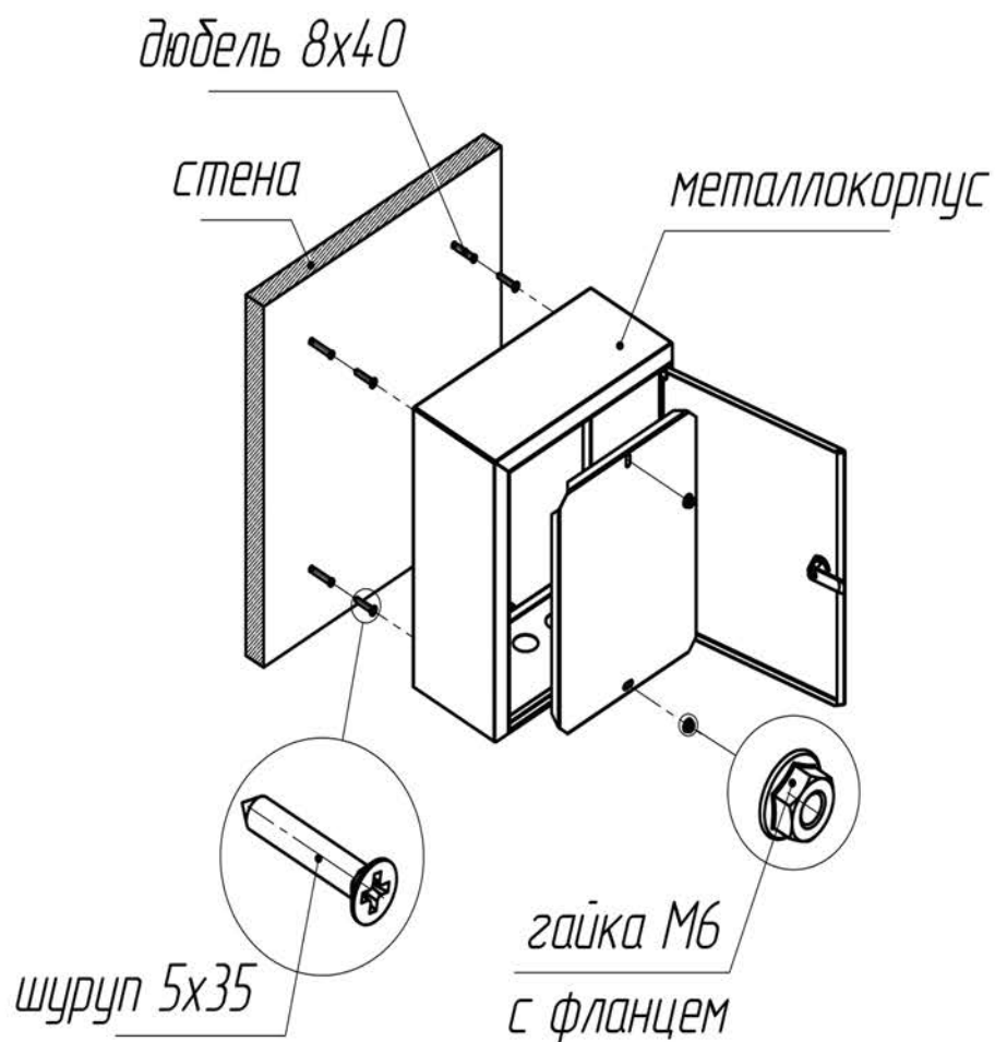
Рис. 1. Схема монтажа
