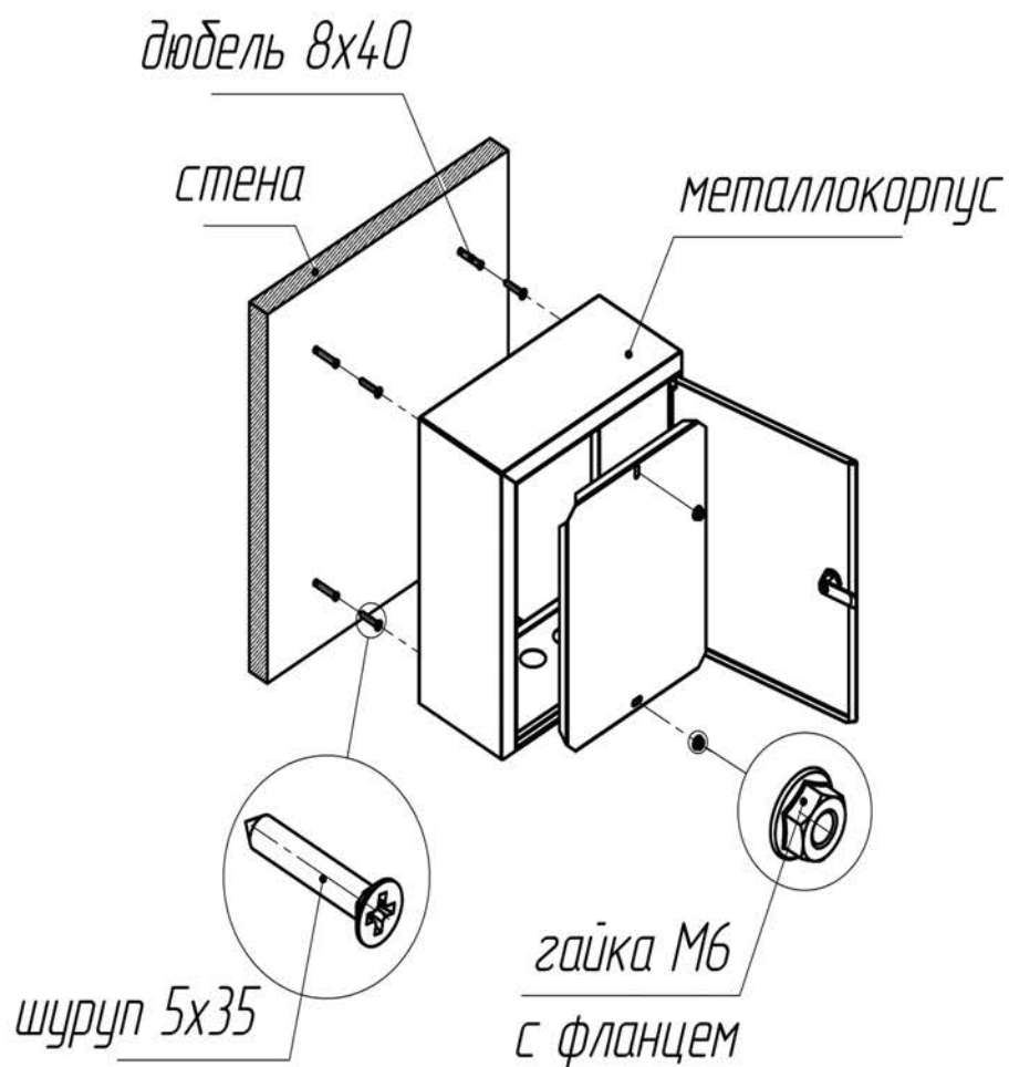
Рис. 1. Схема монтажа
