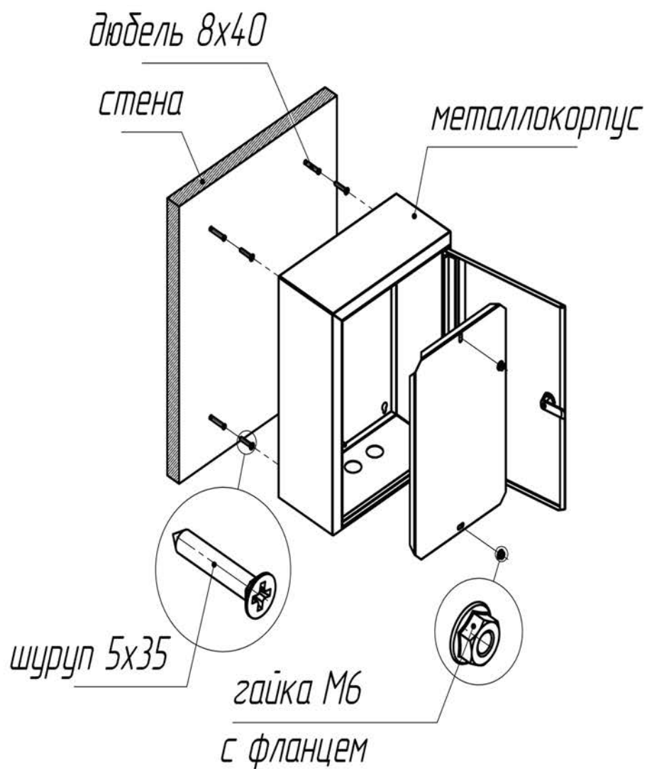
Рис. 1. Схема монтажа
