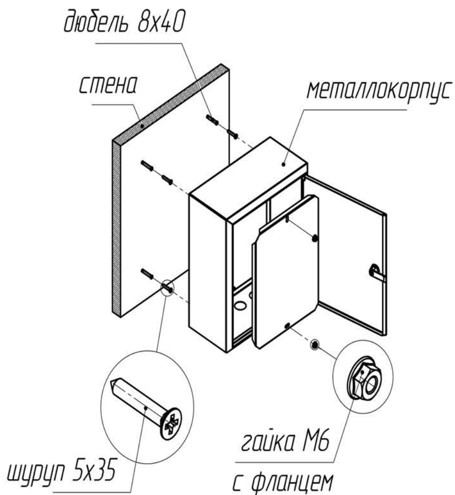
Рис. 1. Схема монтажа
