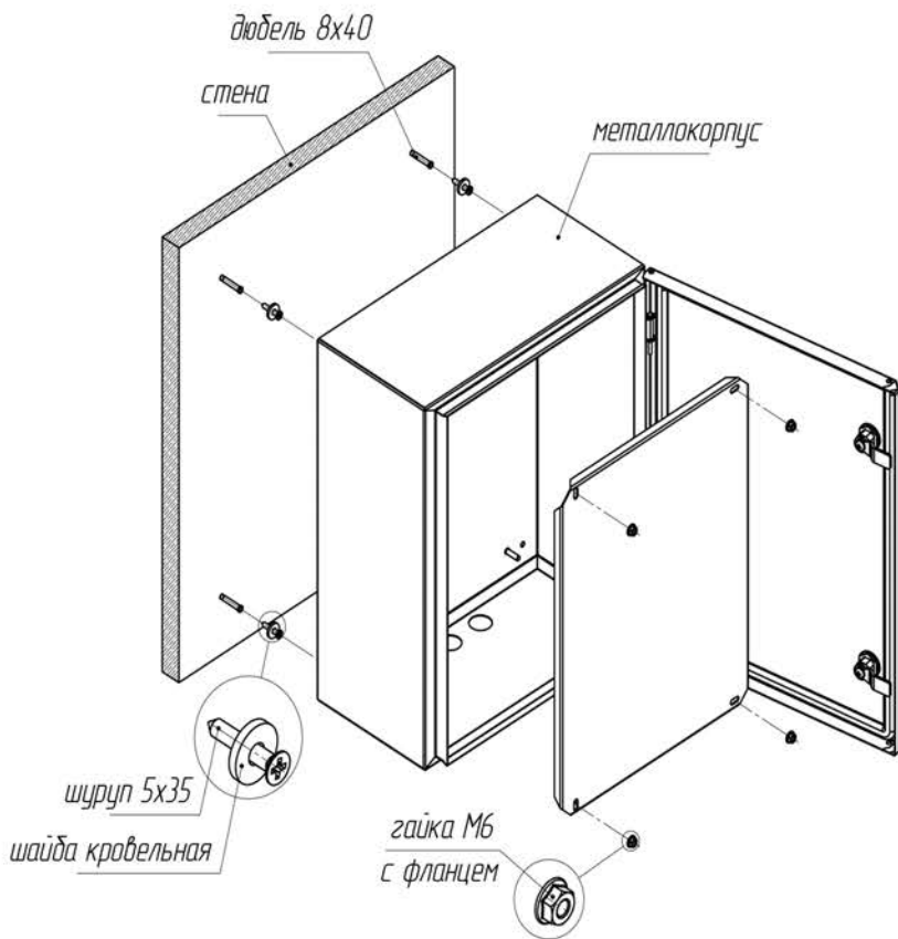
Рис. 1.1 - Схема настенного монтажа
