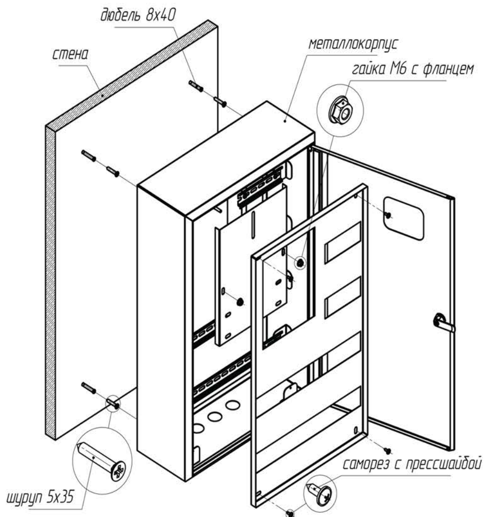
Рис. 1 - Схема монтажа
