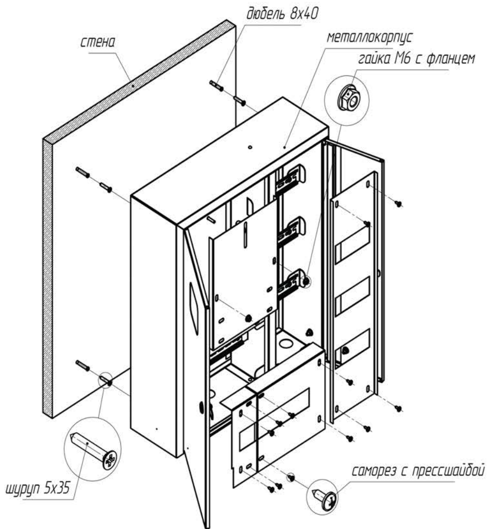
Рис. 1 - Схема монтажа
