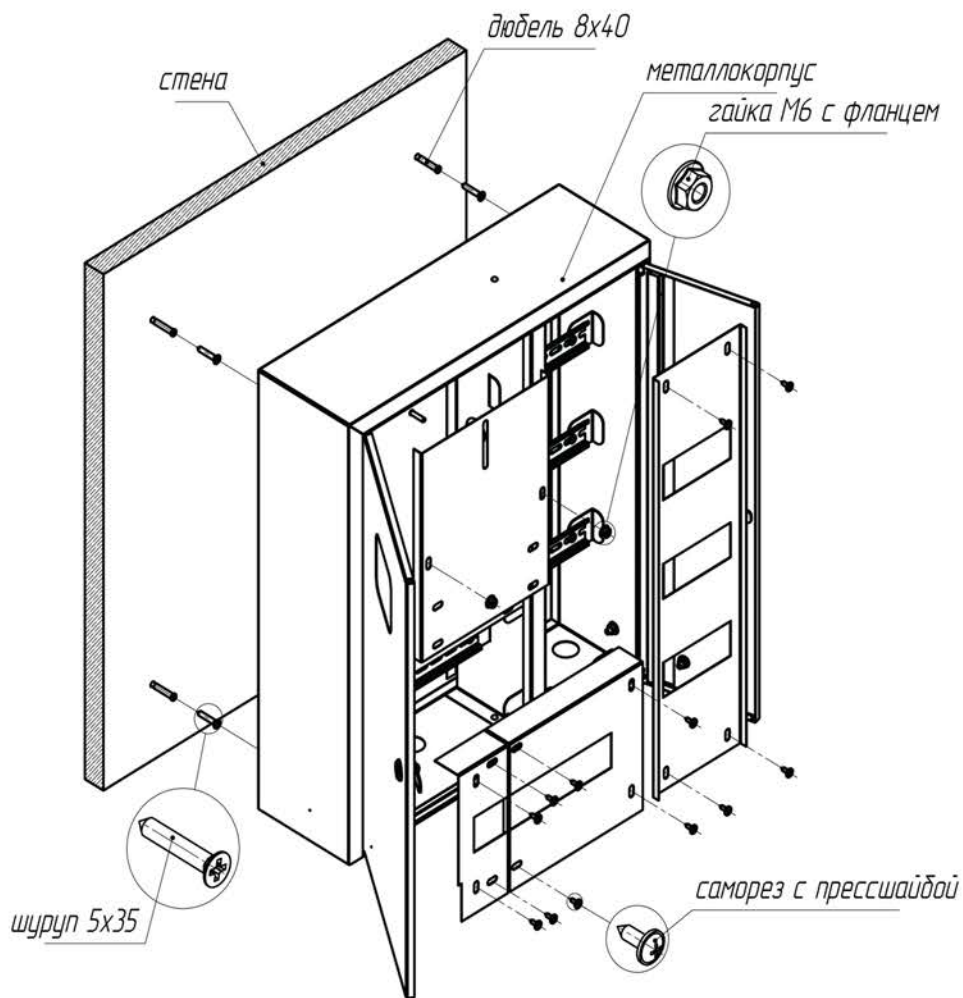
Рис. 1 - Схема монтажа
