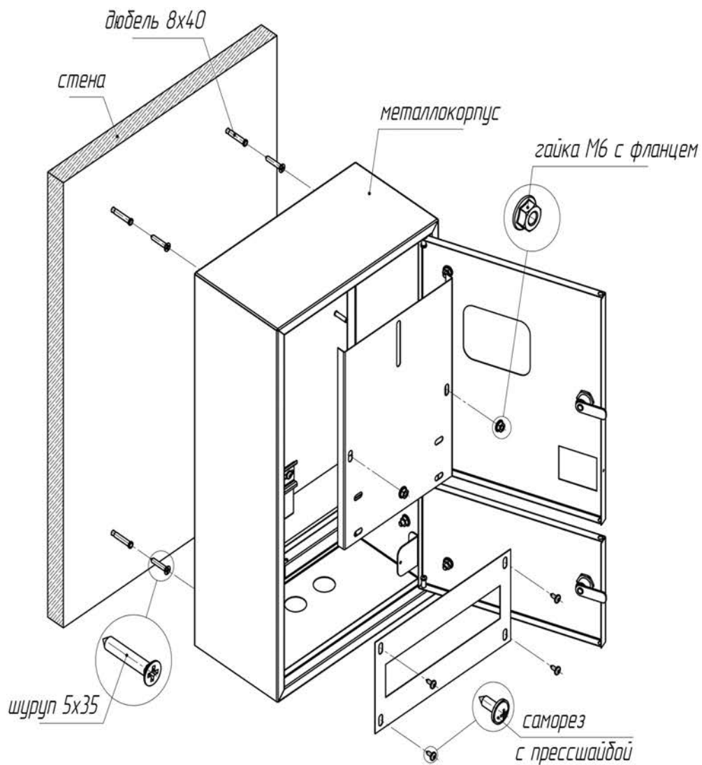
Рис. 1 - Схема монтажа
