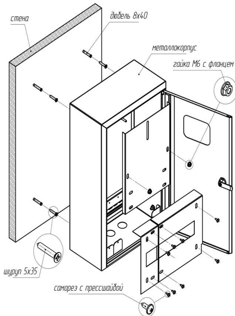
Рис. 1 - Схема монтажа
