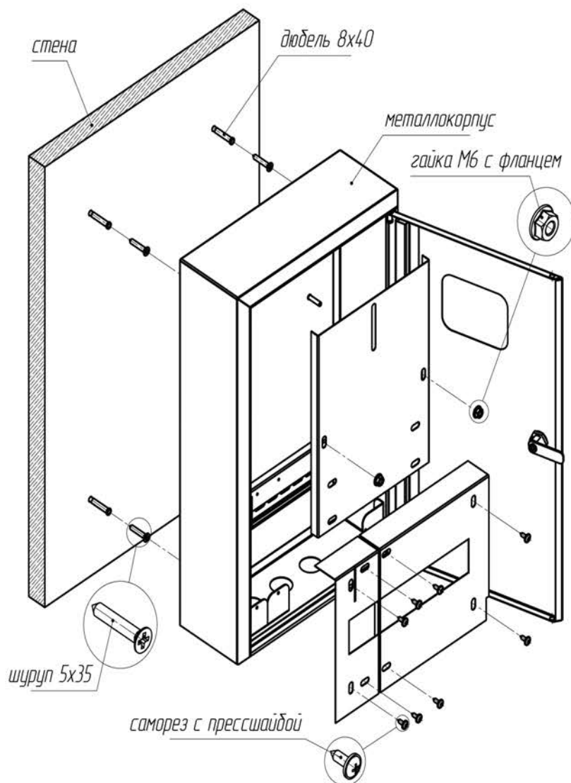
Рис. 1 - Схема монтажа
