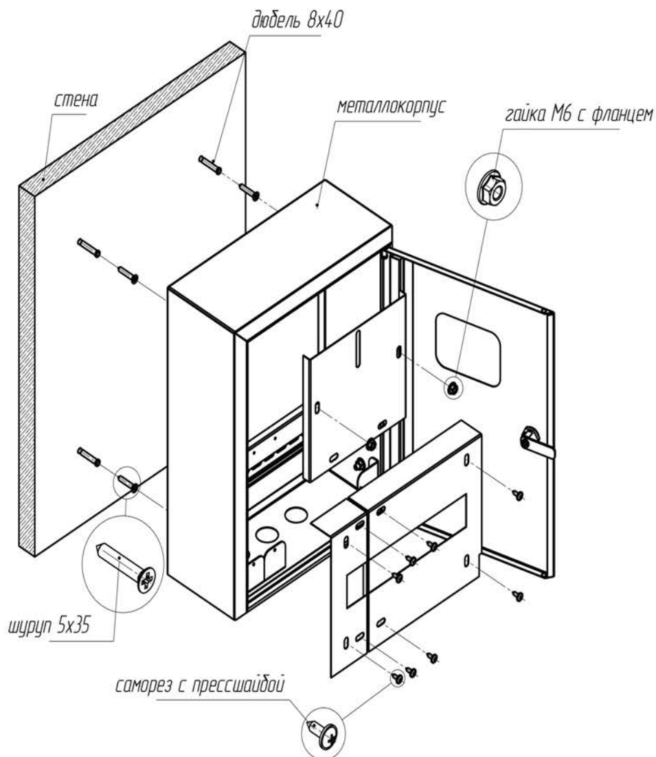
Рис. 1 - Схема монтажа
