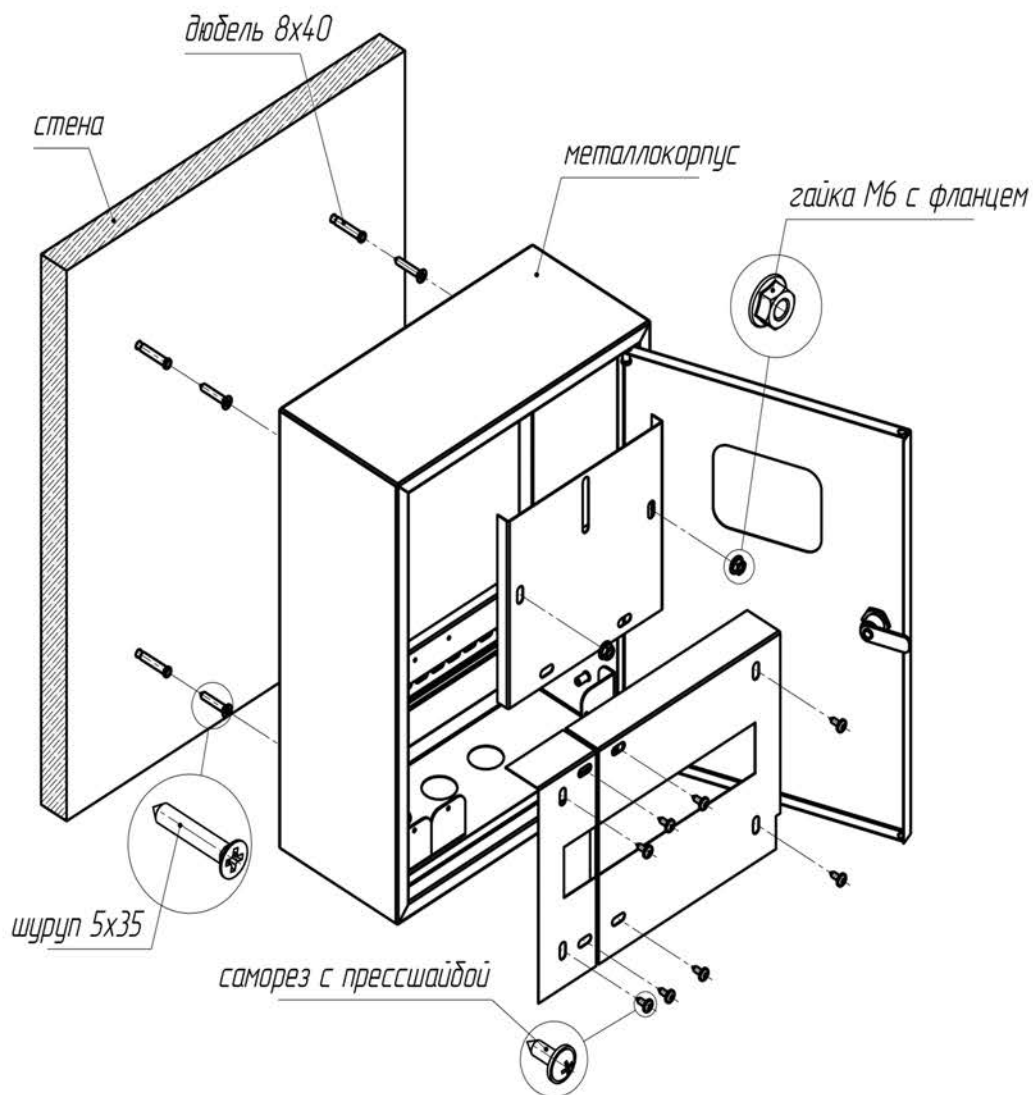
Рис. 1 - Схема монтажа
